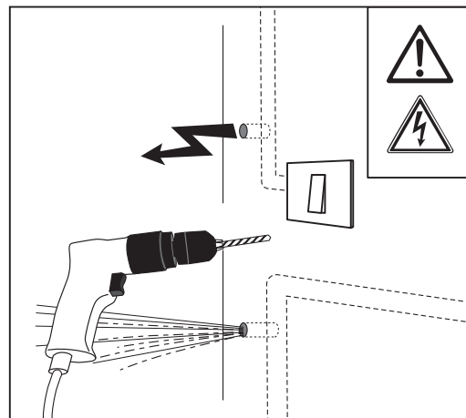
Rischio di folgorazione o esplosione a causa di forature di canalette elettriche o tubazioni con fluidi in pressione (acqua, gas...). Utilizzare un rilevatore di parti metalliche nascoste.
